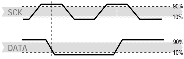
图 12: "启动传输" 时序
